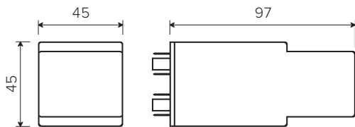
Tutti i relè OK in c.c. e OKUIC con opzione Diode e/o Led
